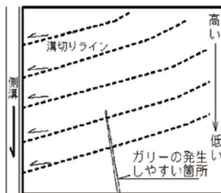
図 1 溝切りの施工例
